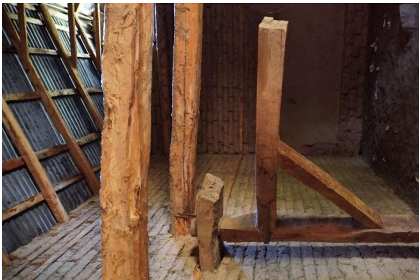
Figura 13. Sistema de regulación del flujo de agua. Molino de Waqar . Foto: AKB.
