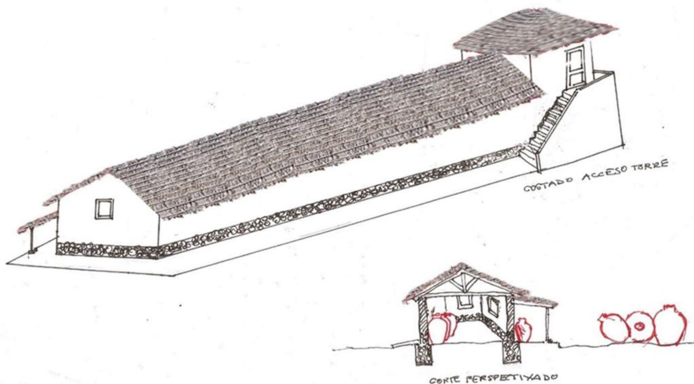
Figura 4. Reconstrucción de la hacienda La Torre con techo de totora. Croquis de la arquitecta Estela Premat; edición y ajustes de AKB.
